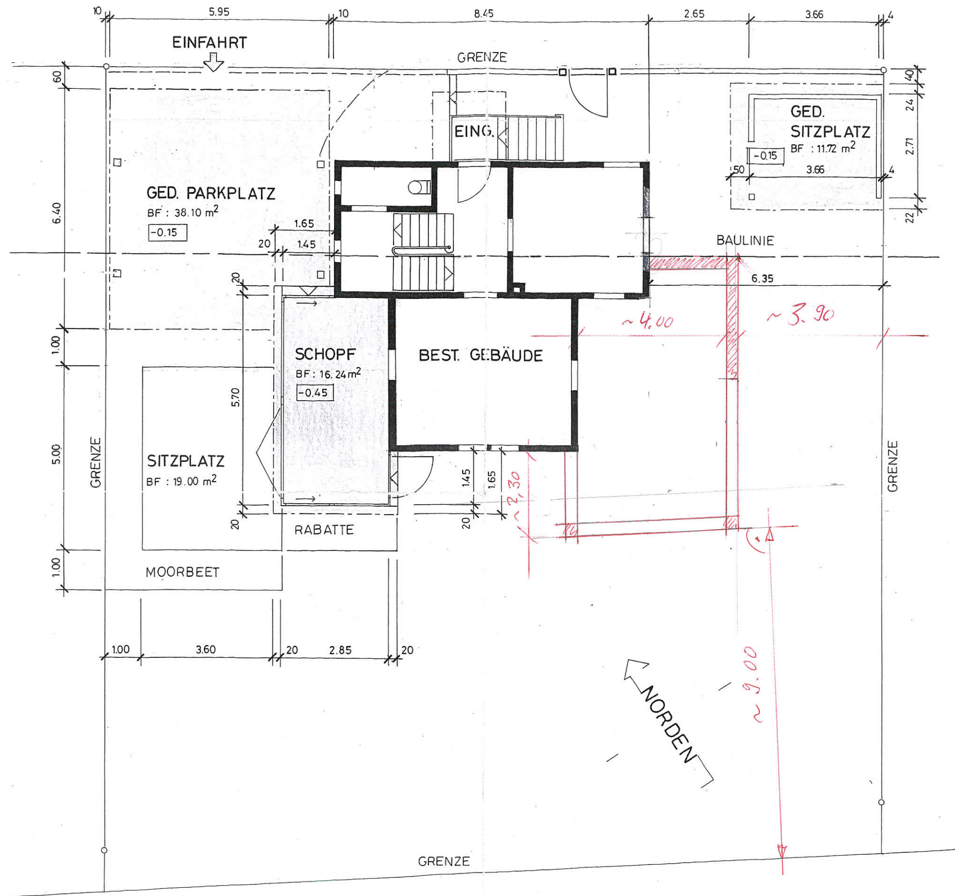
GRUNDRISS MST. 1:100
